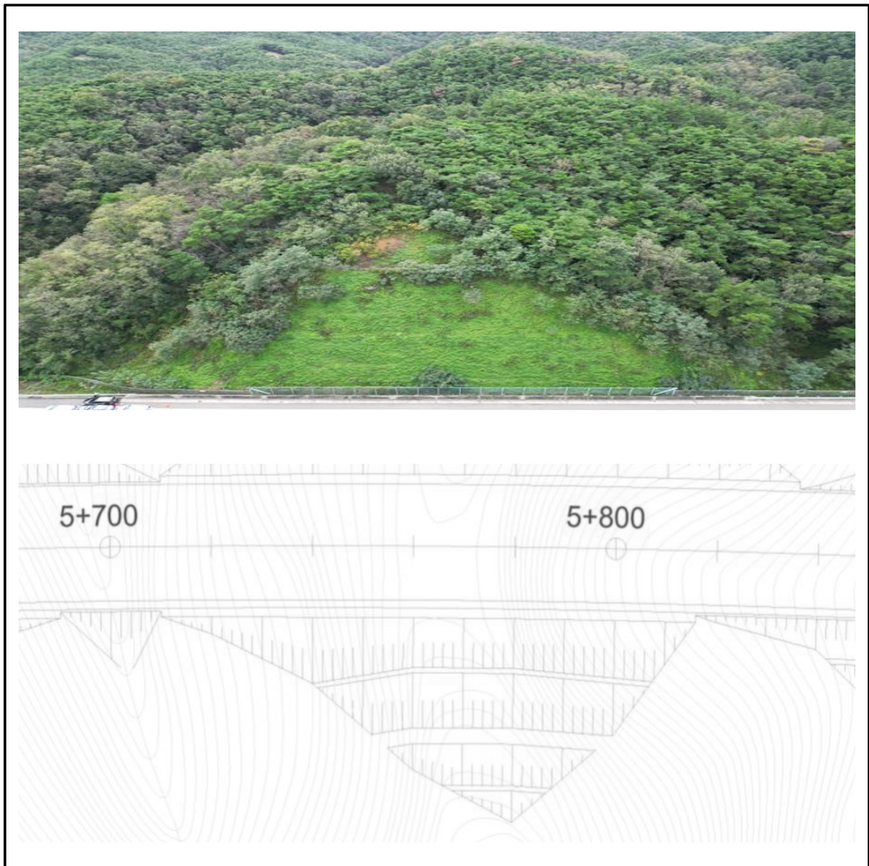
【그림 48.14】 영천절토48 검토대상 비탈면구간
