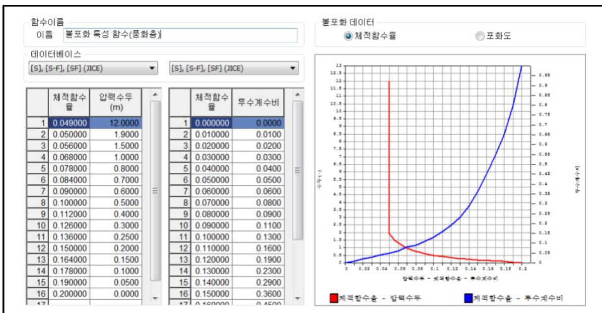
【그림 48.15】 압력수두-채적함수(포화도)-투수계수비 함수
