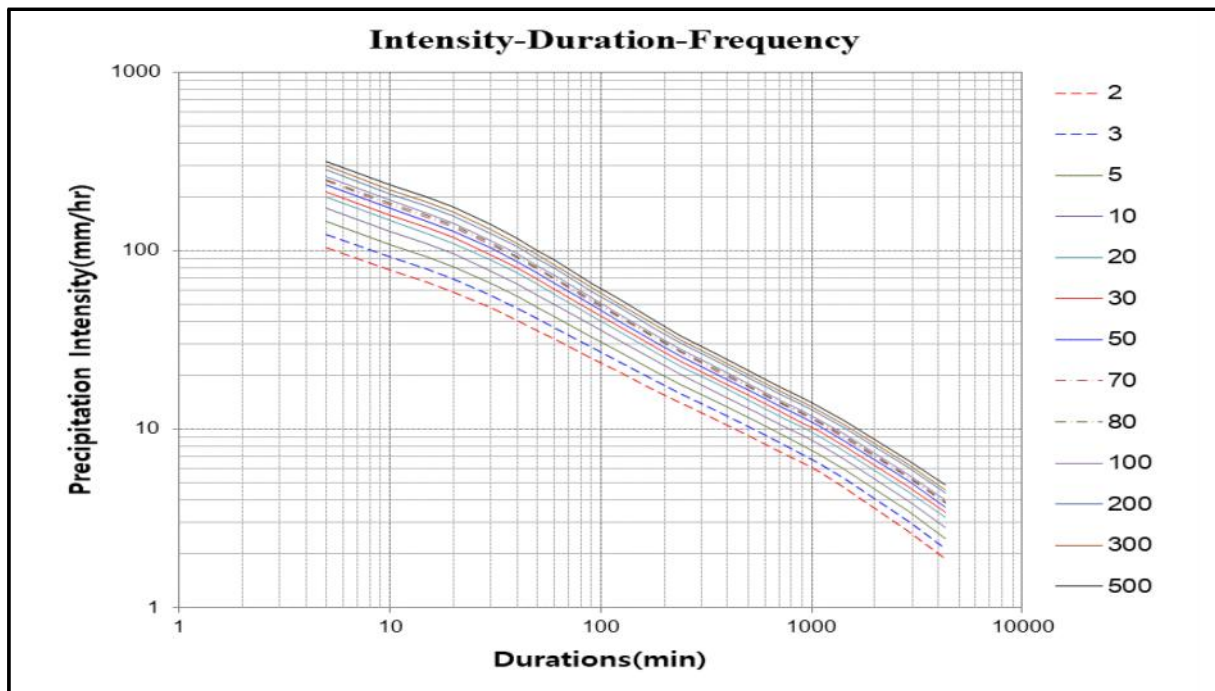
【그림 48.9】 영천지역 IDF곡선
